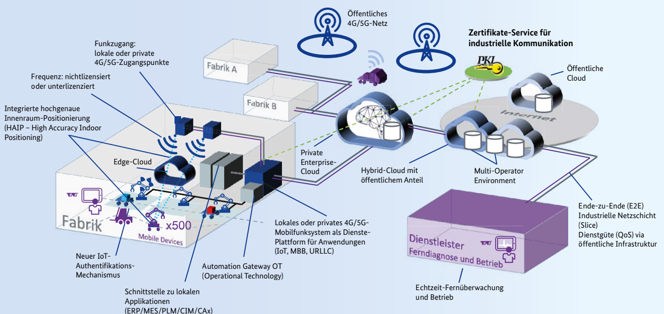
Abbildung 1: Beispiel für Lösungsbausteine eines 5G-Campusnetzes, das im Projekt IC4F betrachtet wird
