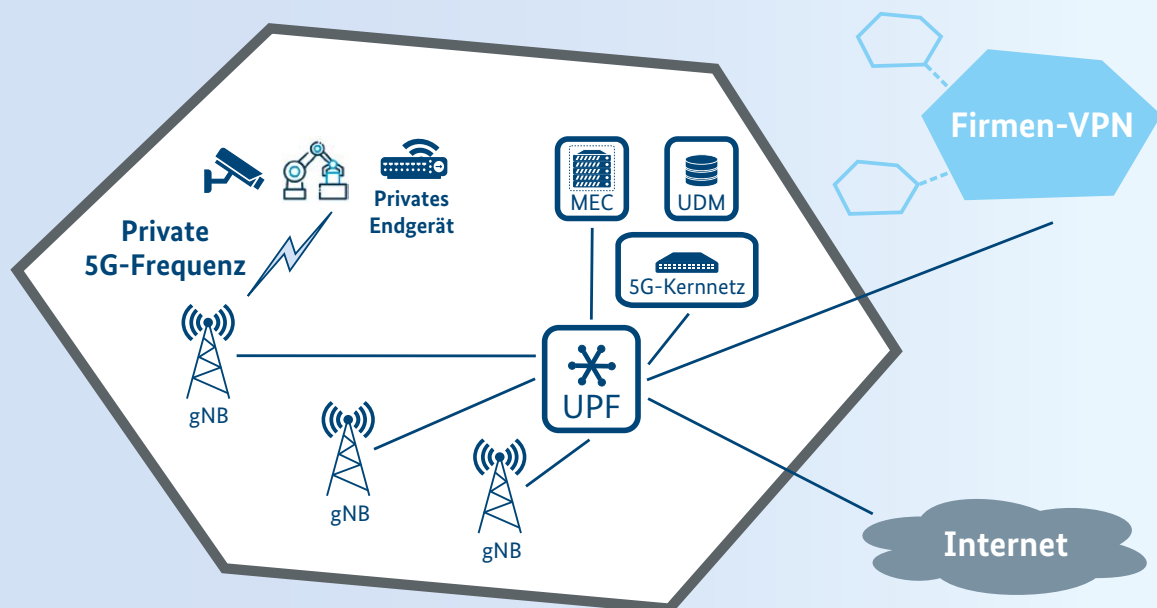
Abbildung 6: Einsatzszenario als separates 5G-Campusnetz (Eigenbetrieb – keine MNO-Integration)
